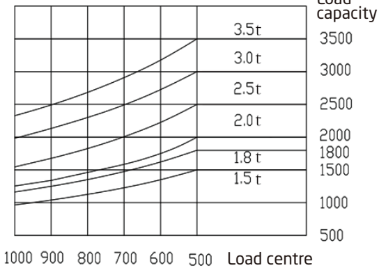
3M duplex mast
